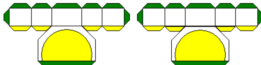
CAIXAS DE RODAS DIANTEIRAS (AS ABAS VERDES SÃO PARA FIXAÇÃO NA CARROCERIA OU NA PLATAFORMA)
