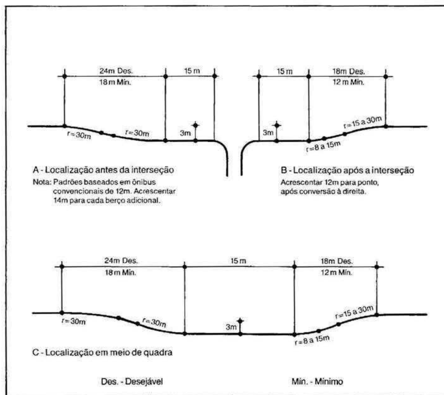
Figura 36 - Localização e dimensões de pontos de parada com reentrância no meio-fio. Fonte: Empresa Metropolitana de Planejamento da Grande São Paulo (22).
